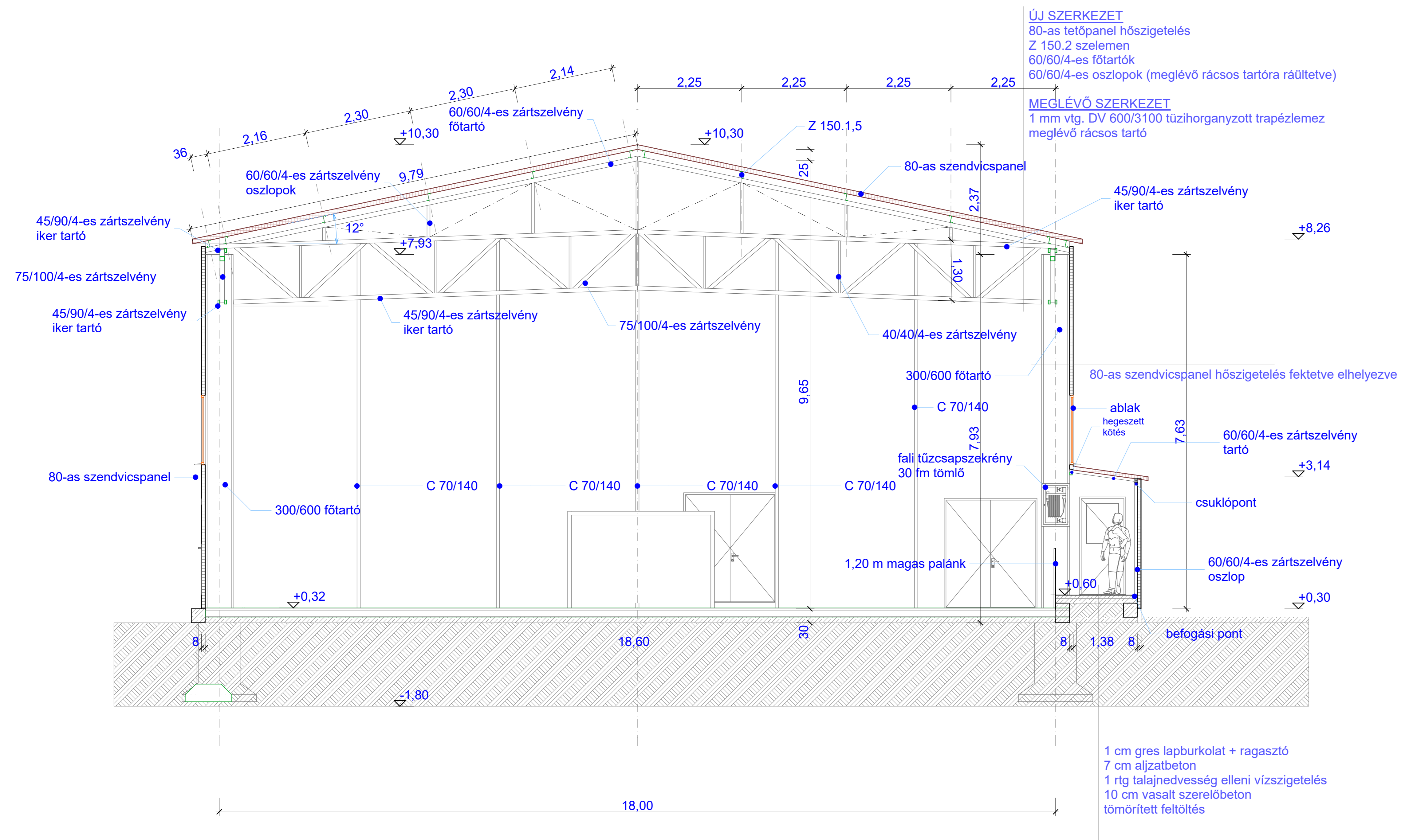
A - A METSZET M = 1 : 100
