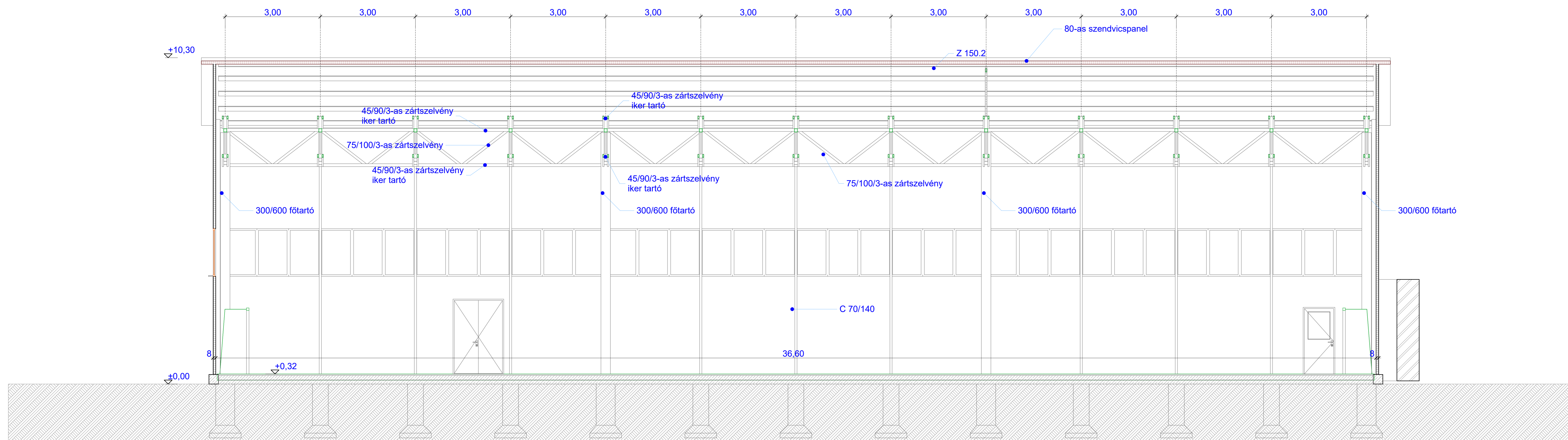
B - B METSZET M = 1 : 100
