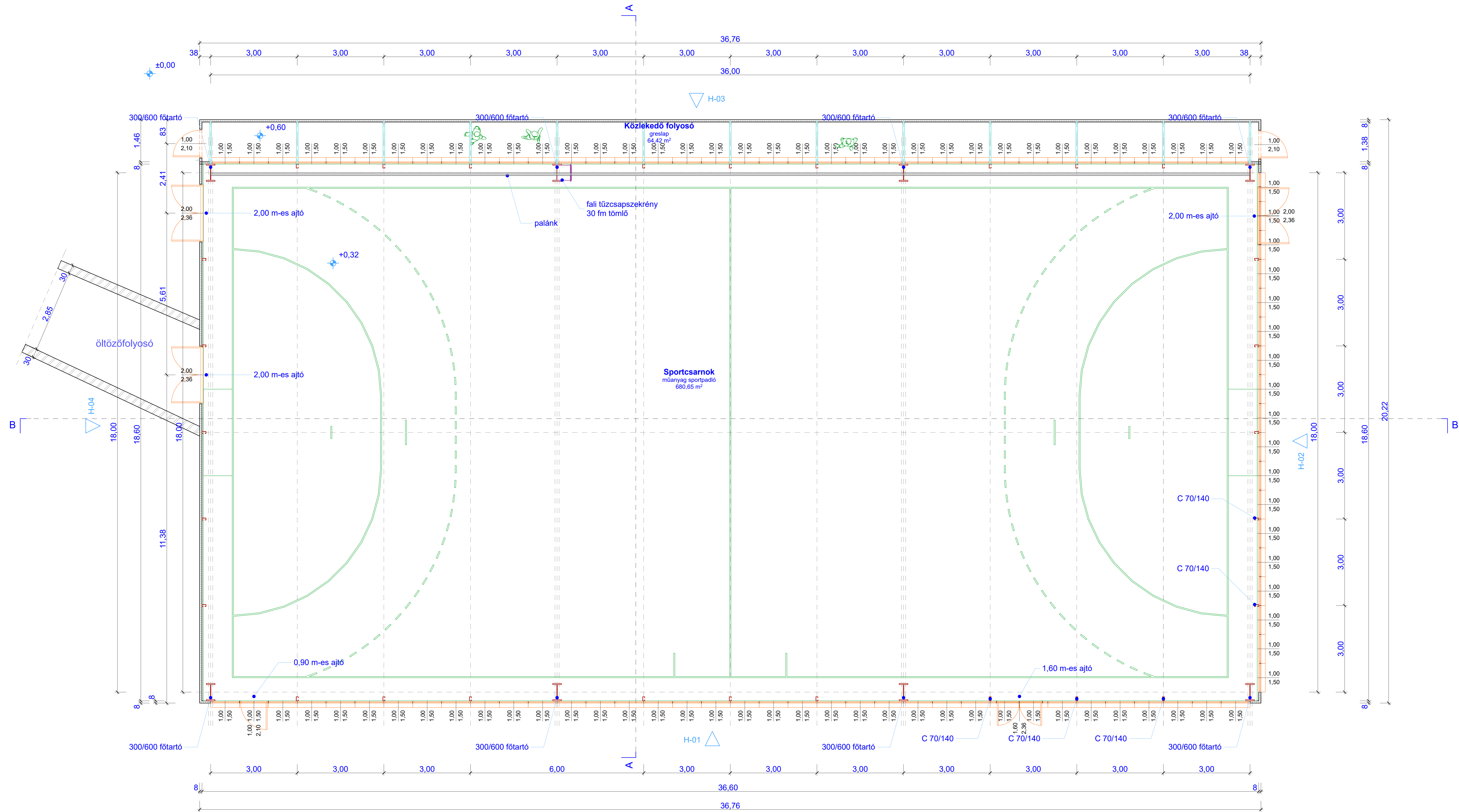
ALAPRAJZ M = 1 : 100
