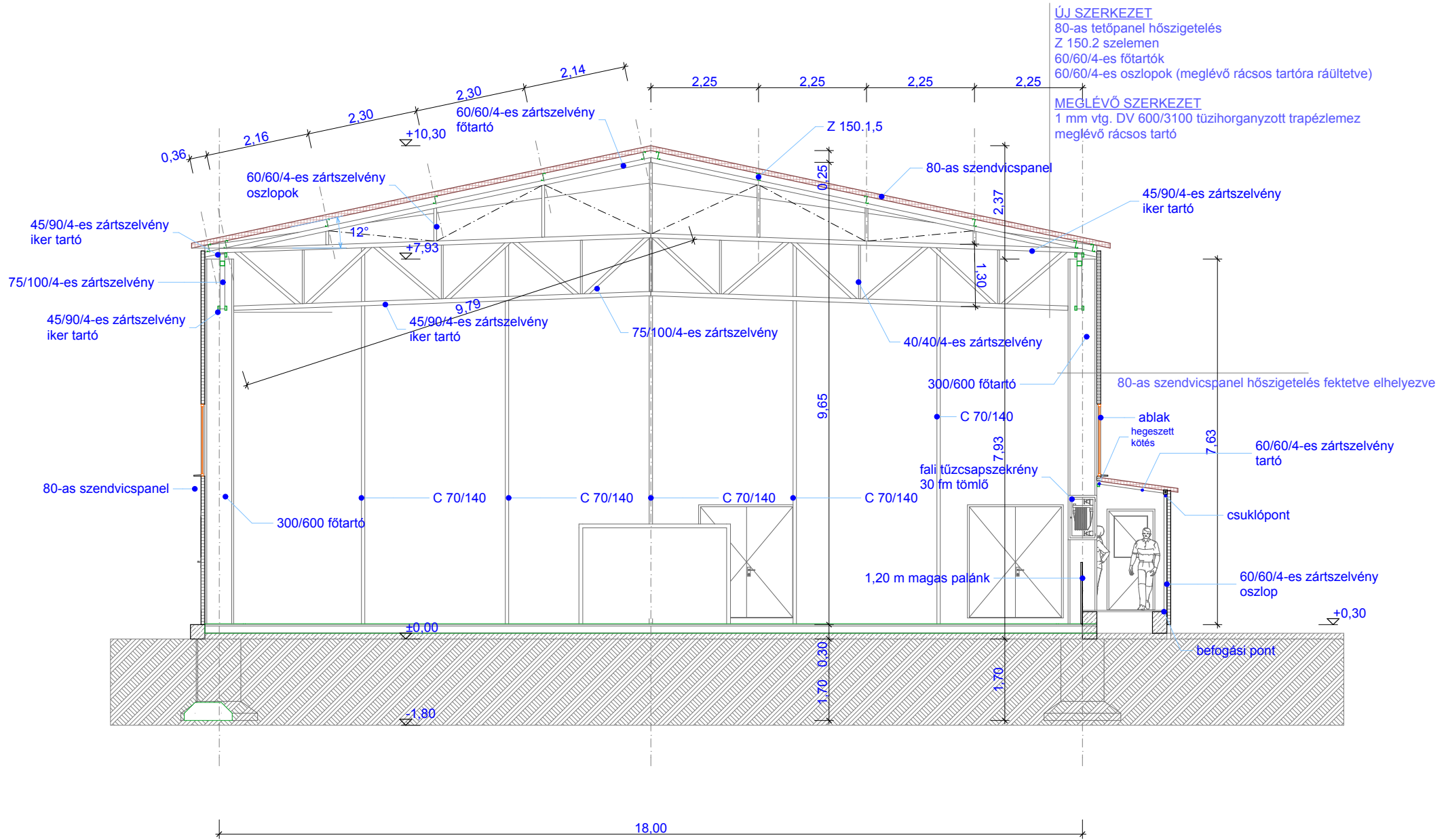
A - A METSZET M = 1 : 100
